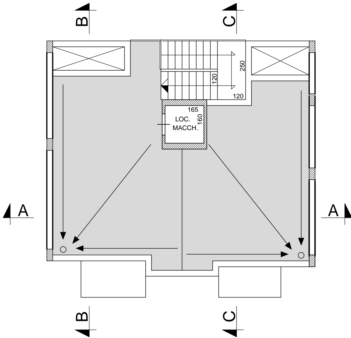
PIANTA PIANO TERRAZZA
