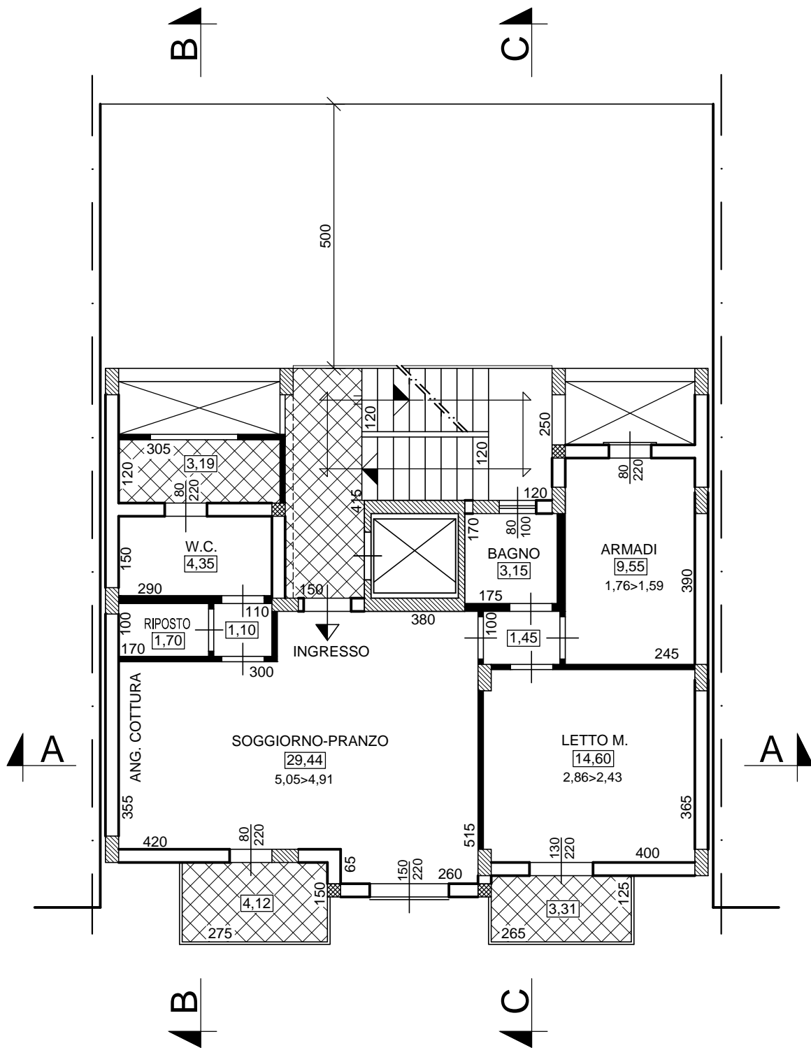
PIANTA PIANO SECONDO E TERZO
